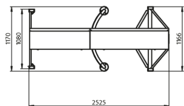
A - A ( 1 : 15 )
